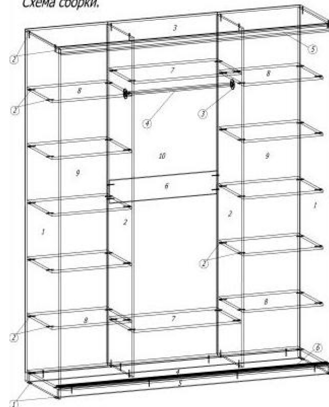
Схема сборки.
